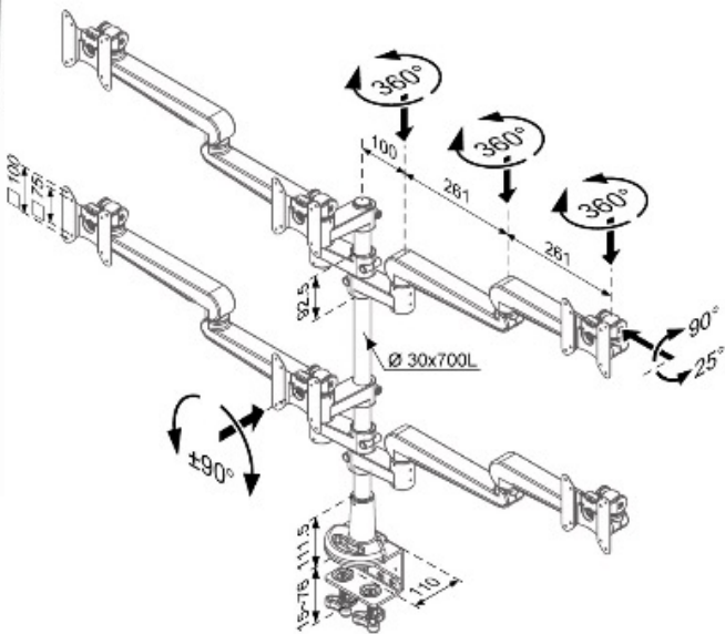
Clamp Type unit:mm
